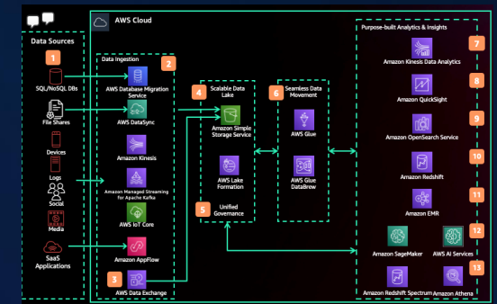
To-Beデータ基盤 (案)
