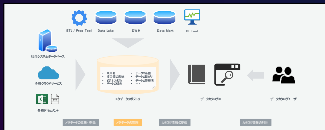
現行データ基盤
